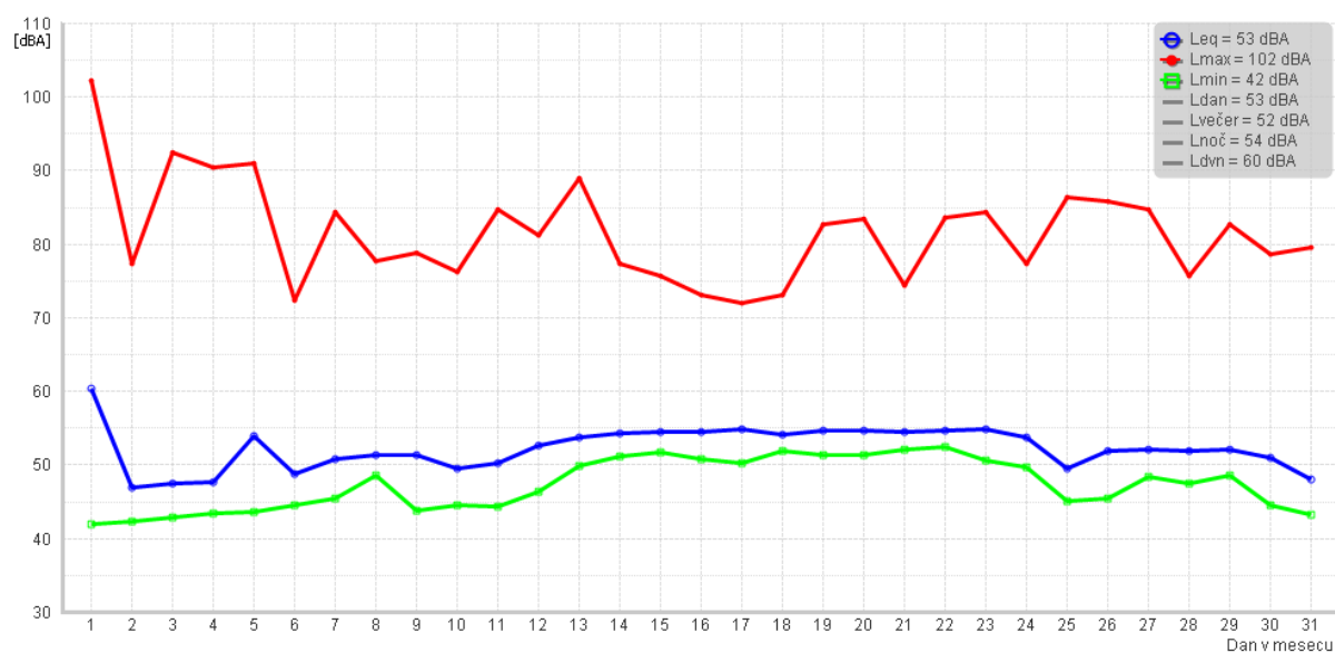
Slika 3: Urne vrednosti za obdobje od 01.01.2015 do 31.01.2015
