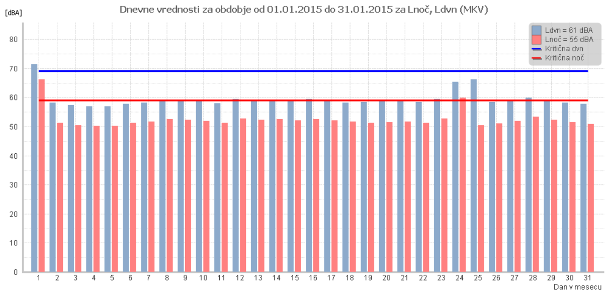
Slika 11: Dnevne vrednosti za obdobje od 01.01.2015 do 31.01.2015 za L_{noč} in L_{dvn} (MKV)
