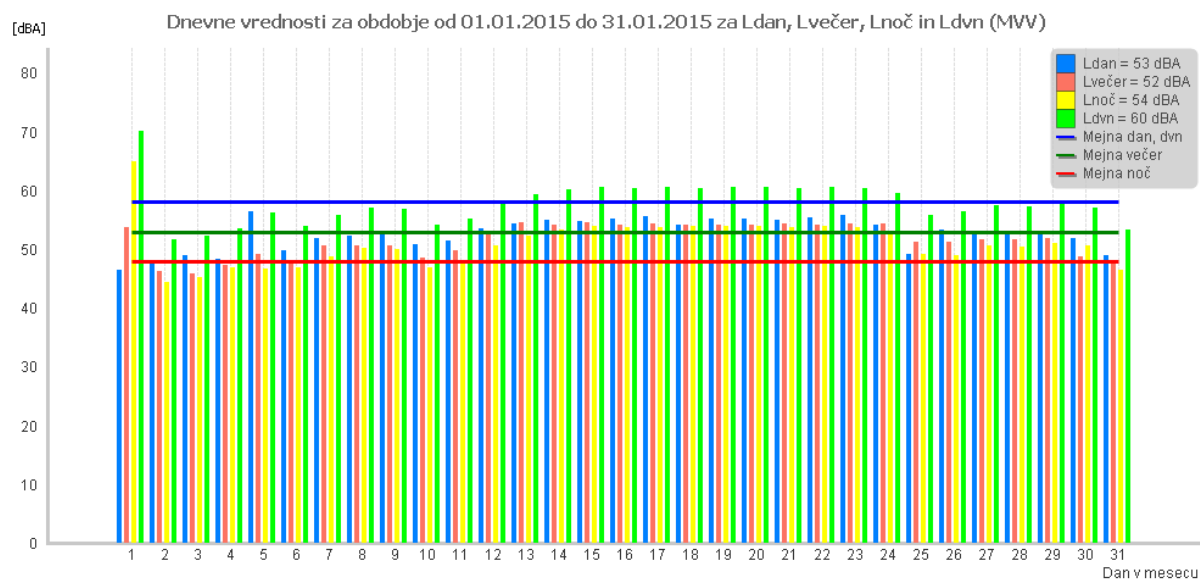
Slika 6: Dnevne vrednosti za obdobje od 01.01.2015 do 31.01.2015 za L_{dan} , L_{večer} , L_{noč} in L_{dvn} (MVV)
