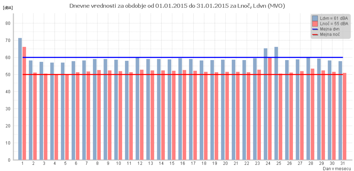
Slika 10: Dnevne vrednosti za obdobje od 01.01.2015 do 31.01.2015 za L_{noč} in L_{dvn} (MVO)
