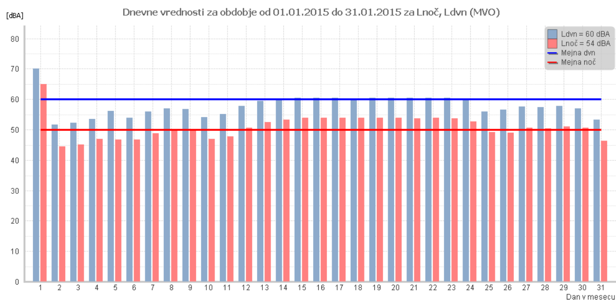
Slika 4: Dnevne vrednosti za obdobje od 01.01.2015 do 31.01.2015 za L_{noč} in L_{dvn} (MVO)
