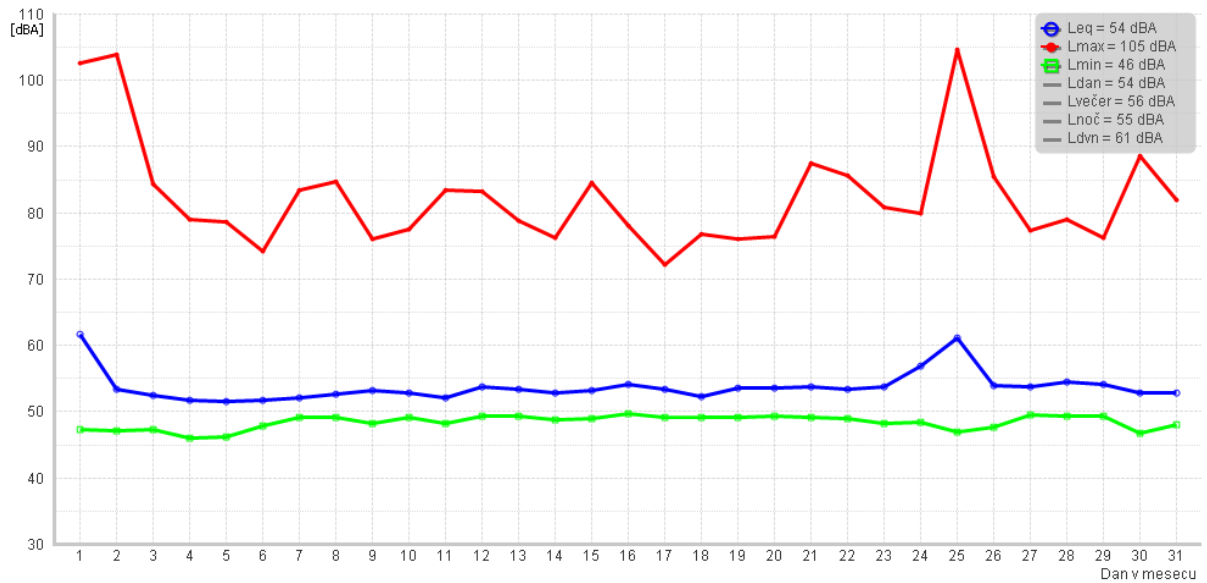
Slika 9: Urne vrednosti za obdobje od 01.01.2015 do 31.01.2015
