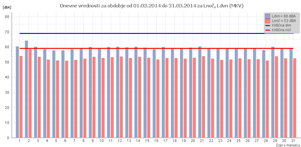
Slika 11: Dnevne vrednosti za obdobje od 01.03.2014 do 31.03.2014 za L_{noč} in L_{dvn} (MKV)
