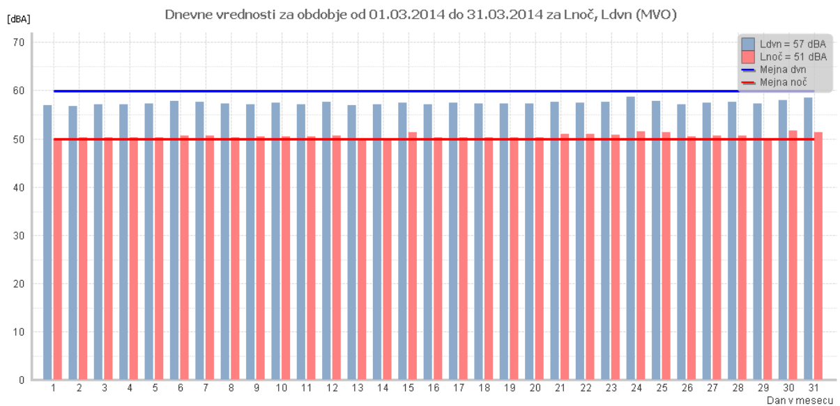
Slika 4: Dnevne vrednosti za obdobje od 01.03.2014 do 31.03.2014 za L_{noč} in L_{dvn} (MVO)
