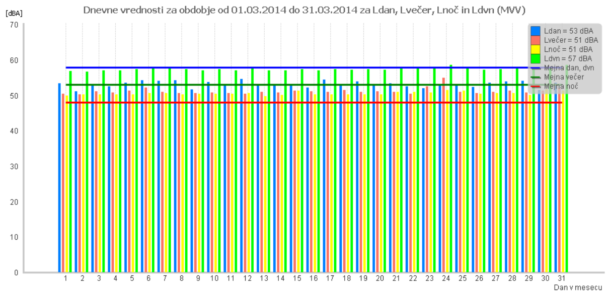
Slika 6: Dnevne vrednosti za obdobje od 01.03.2014 do 31.03.2014 za L dan , L večer , L noč in L dvn (MVV)
