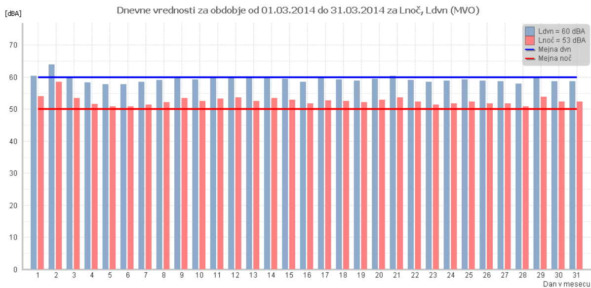
Slika 10: Dnevne vrednosti za obdobje od 01.03.2014 do 31.03.2014 za L noč in L dvn (MVO)
