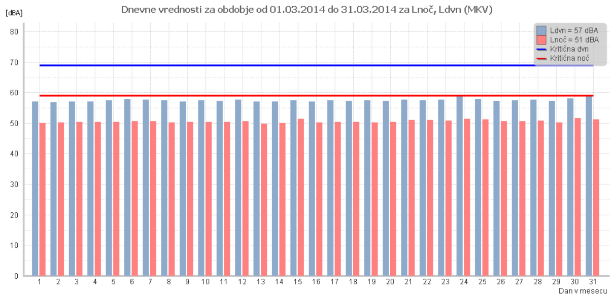
Slika 5: Dnevne vrednosti za obdobje od 01.03.2014 do 31.03.2014 za L noč in L dvn (MKV)
