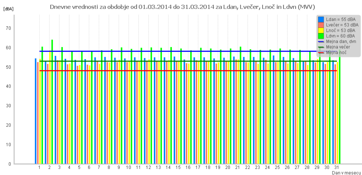
Slika 12: Dnevne vrednosti za obdobje od 01.03.2014 do 31.03.2014 za L_{dan} , L_{večer} , L_{noč} in L_{dvn} (MVV)
