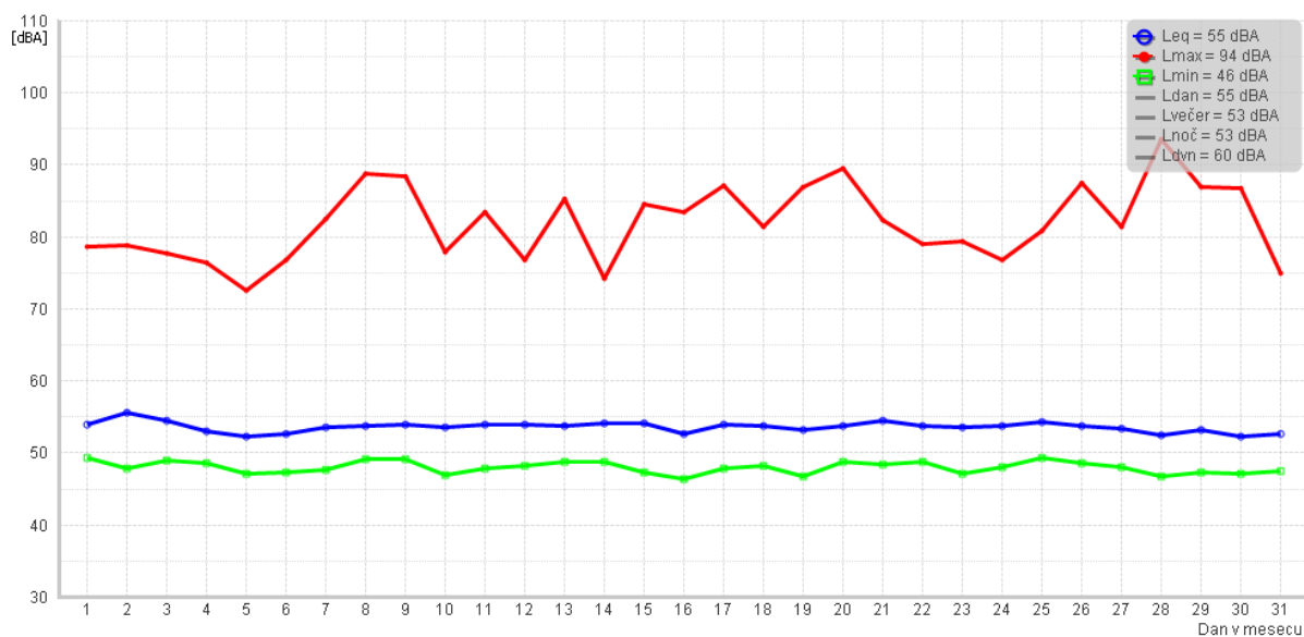
Slika 9: Urne vrednosti za obdobje od 01.03.2014 do 31.03.2014
